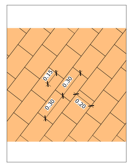
Pflasterformat 20 / 30 im Läuferverband
