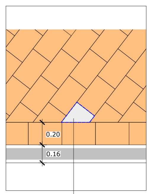
Schnittkante am geraden Randbereich
