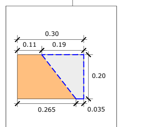
Mindestgröße Schlussstein am Pflasterstreifen
