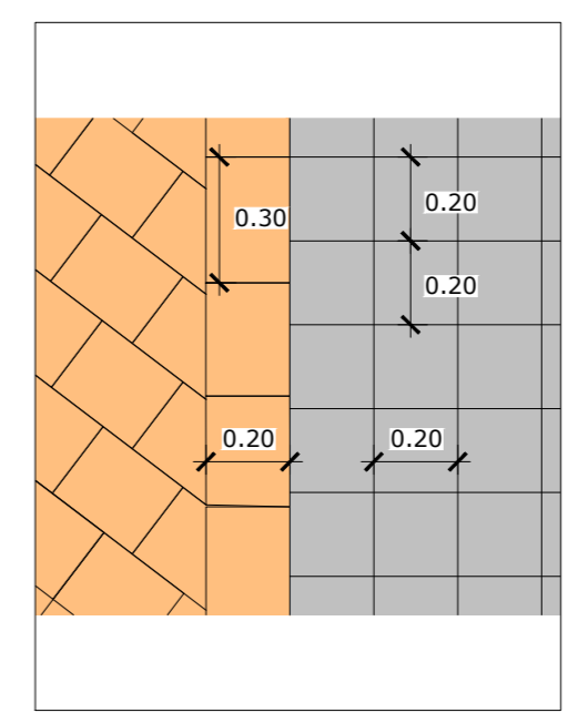
Übergang Fahrbahn / PKW-Stellplatz
